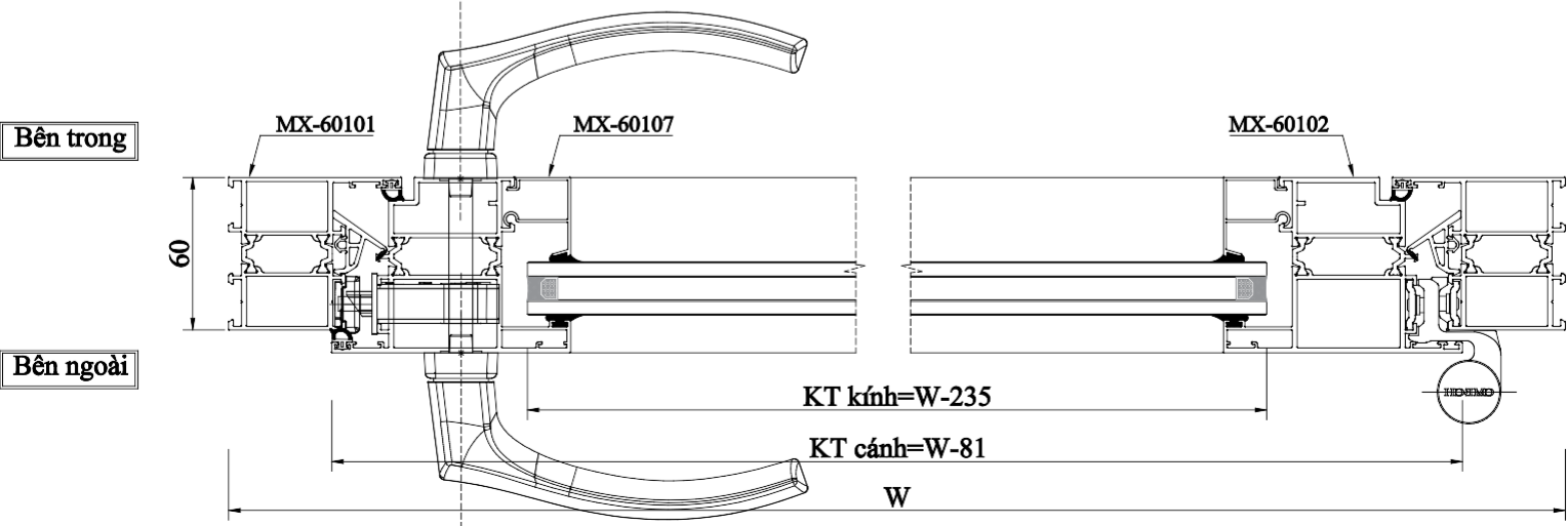
Mặt cắt 2-2
